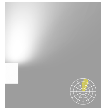
ARO2 3 Asymmetric Refractive Optic
